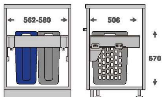
JD04H-600 CESTO DUAL PARA ROPA (CON CORREDERA CIERRE SUAVE)
